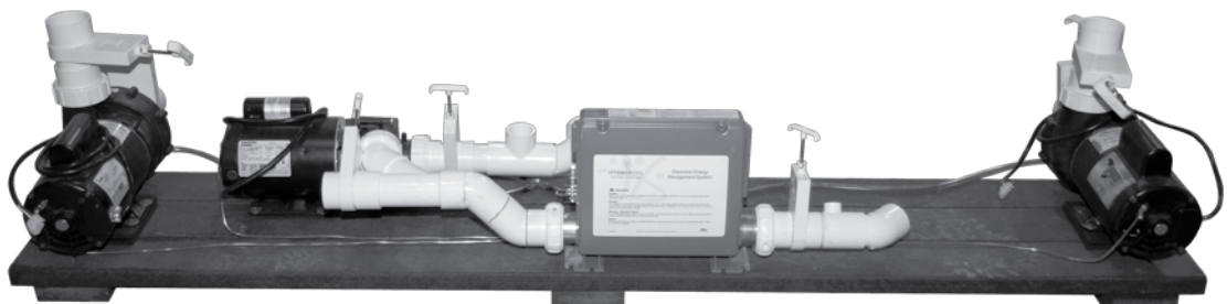
PLATE-FORME POUR ÉQUIPEMENT DE FONCTIONNEMENT AQUASPORT – TYPIQUE (VERSION NORD-AMÉRICAIN ILLUSTRÉE)
