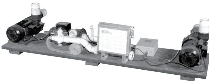
PLATE-FORME POUR ÉQUIPEMENT DE FONCTIONNEMENT AQUASPORT – TYPIQUE (VERSION NORD-AMÉRICAIN ILLUSTRÉE)
